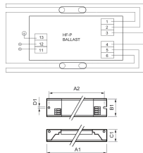
Technische Daten Philips HF-P 254/255 TL5 HO/PLL III 220-240V IDC
